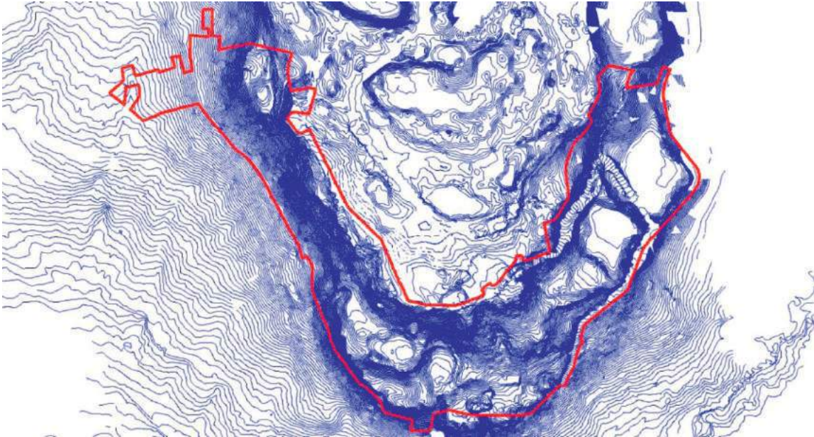
Resim 4: Eğim Haritası
