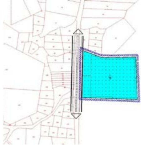
Resim 3: Öneri 1/1000 Ölçekli Uygulama İmar Planı
