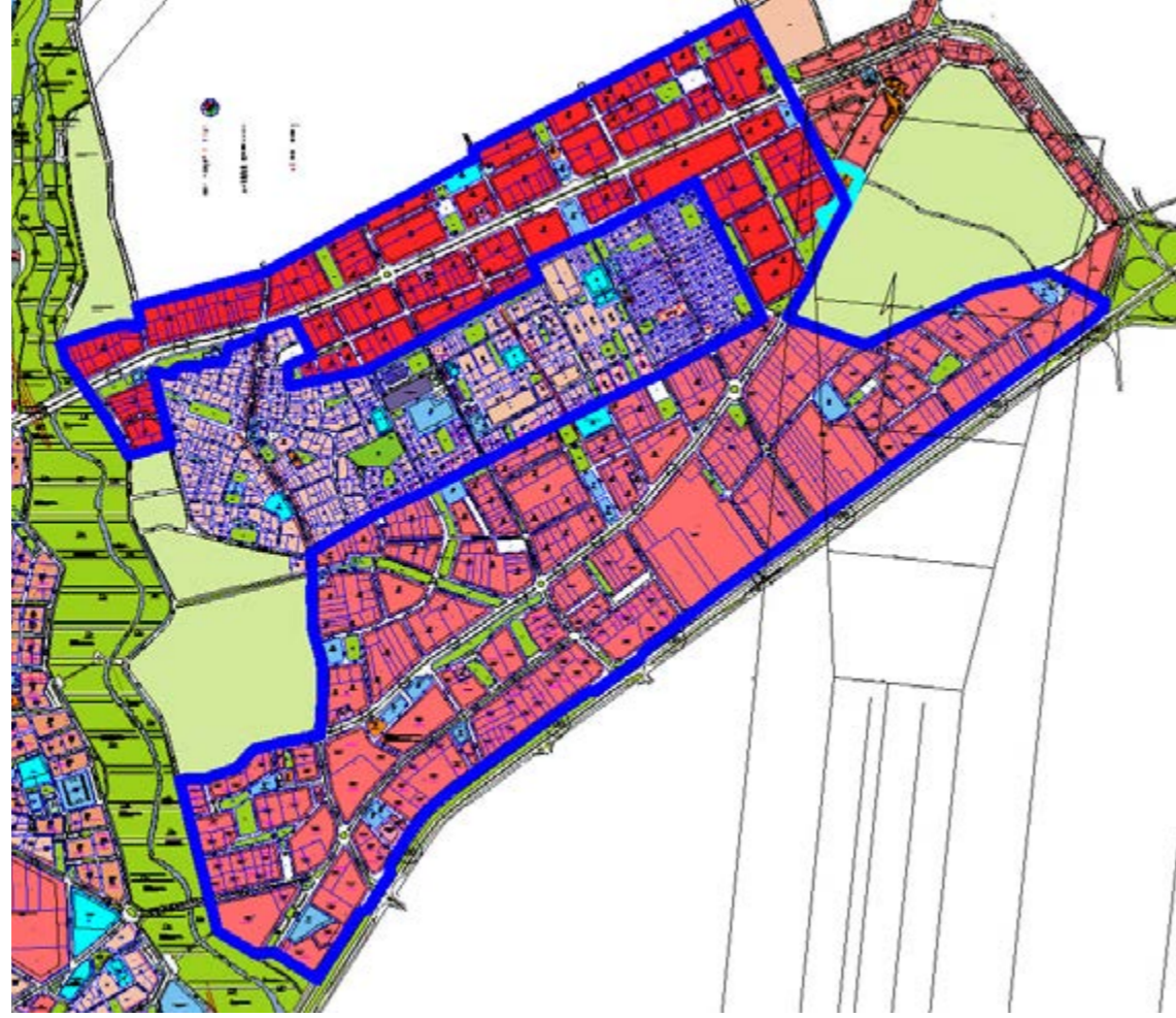
Resim 3: Öneri 1/1000 Ölçekli Uygulama İmar Planı
