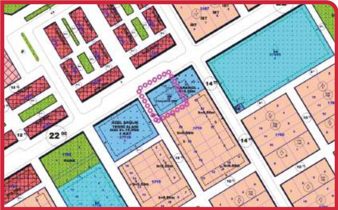
Resim 4: Öneri 1/1000 Ölçekli Uygulama İmar Planı
