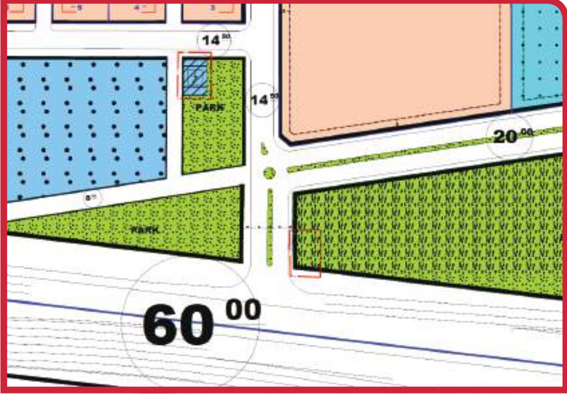
Resim 5: öneri Uygulama İmar Planı
