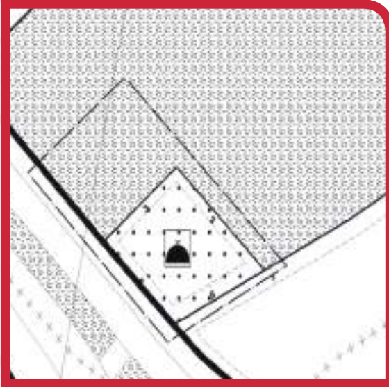
Resim 2: mevcut 1/1000 Ölçekli Uygulama İmar Planı
