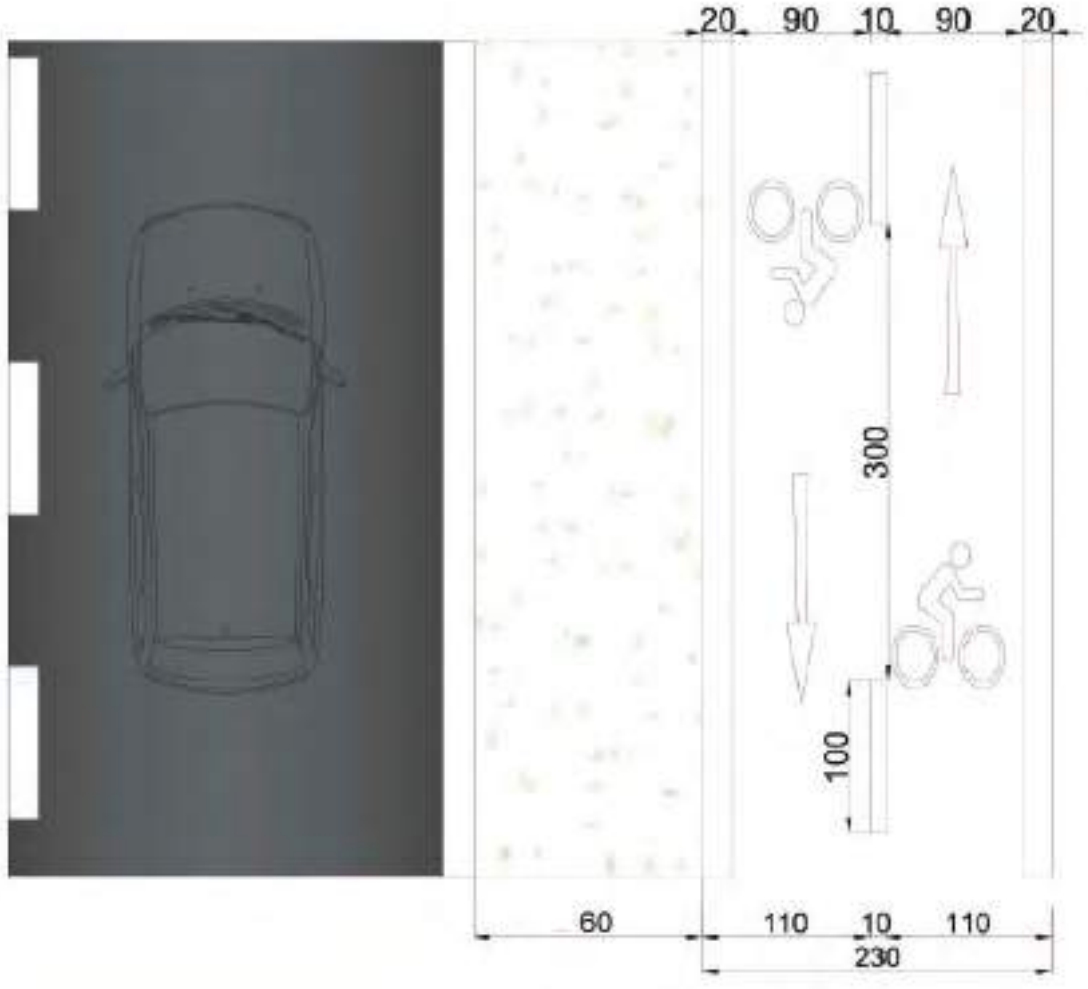
Resim 4 : Çift Yönlü Bisiklet Yolu Bandı Kesiti
