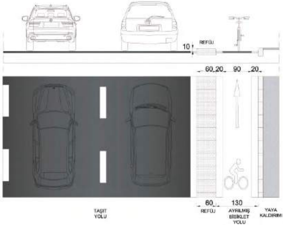
Resim 3: Tek Yönlü Bisiklet Yolu Bandı Kesiti
